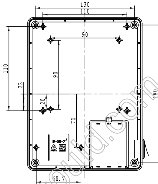
下盖正视图
