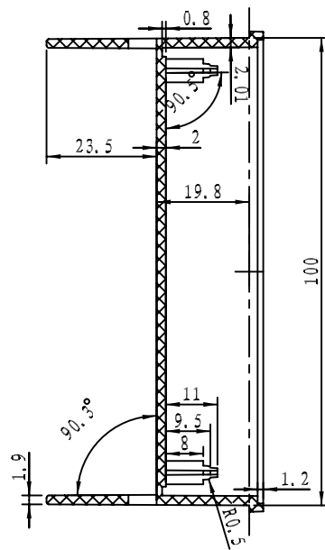
剖面 A-A
