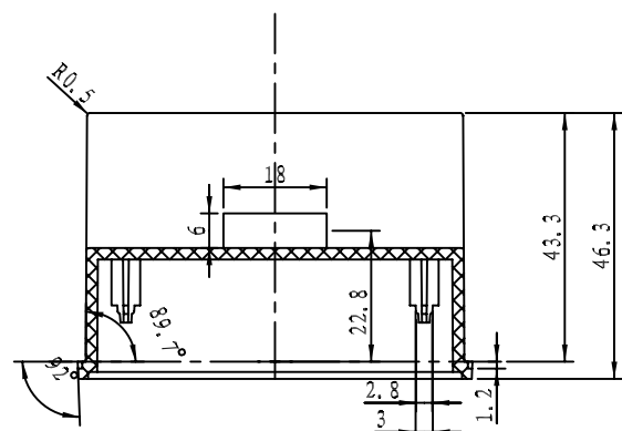
剖面 B-B
