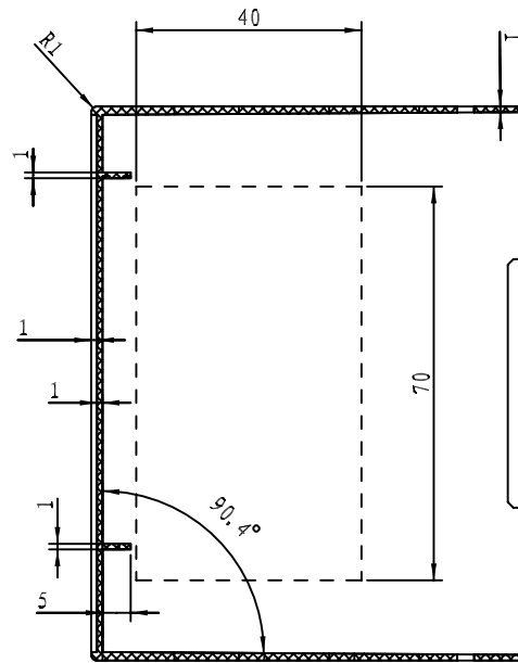
剖面 A-A
