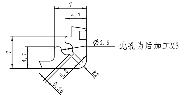
细节 A 比例 3:1
