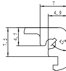
细节 B 比例 3:1
