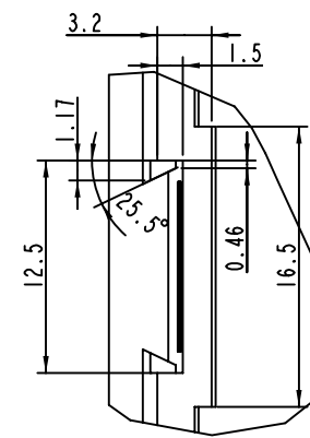
细节 B 比例 3:1
