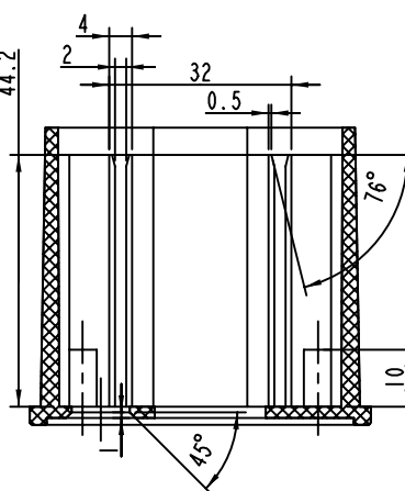
剖面 H-H
