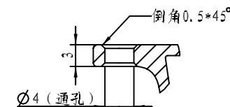
细节 C 比例 2:1
