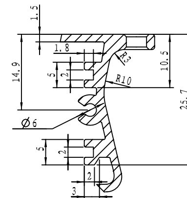
细节 A 比例 2:1
