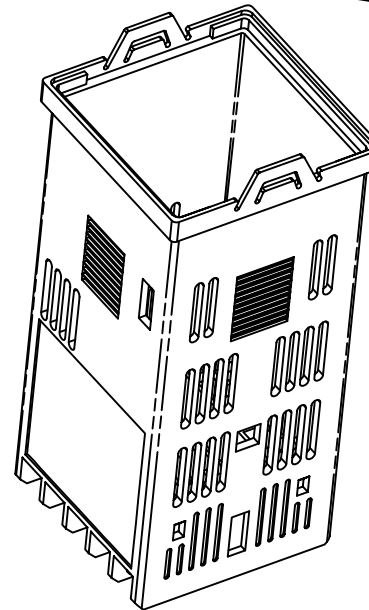
细节 F 比例 3:1
