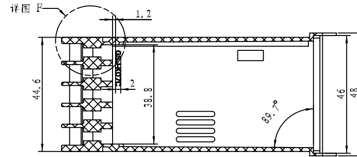
剖面 G-G
