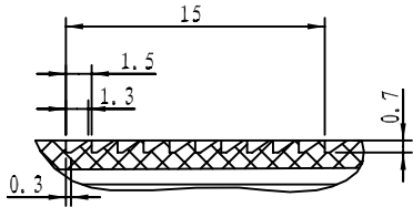
细节 G 比例 3:1
