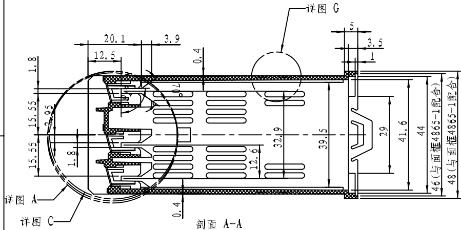
剖面 A-A
