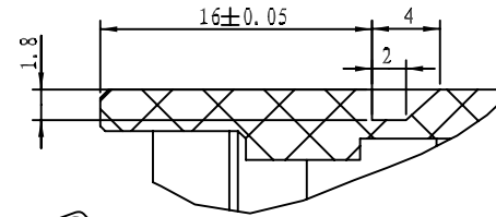
细节 F 比例 3:1
