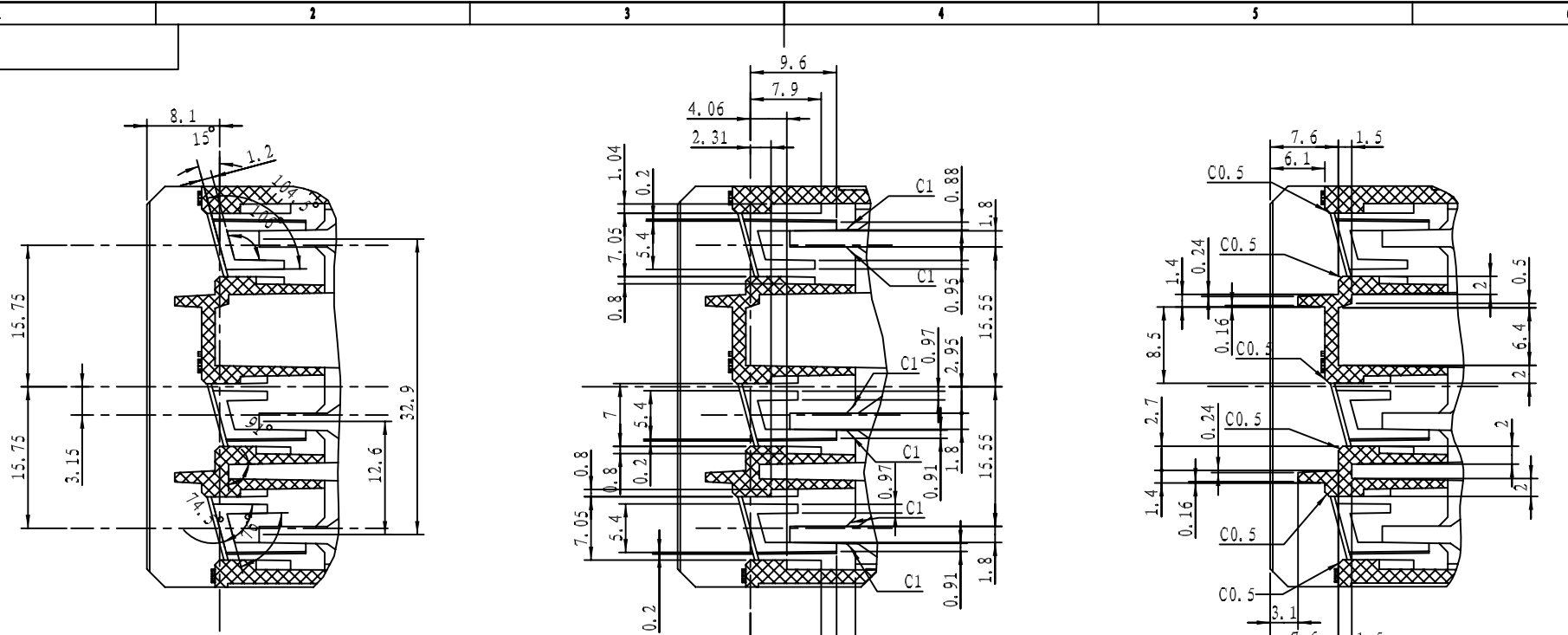
细节 A 比例 2:1
