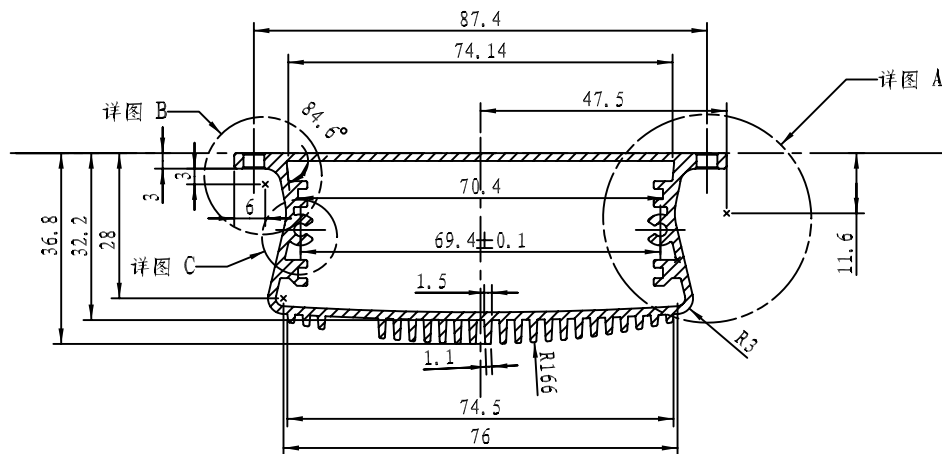
剖面 A-A
