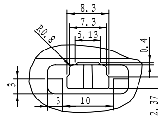
细节 D 刻度 2:1
