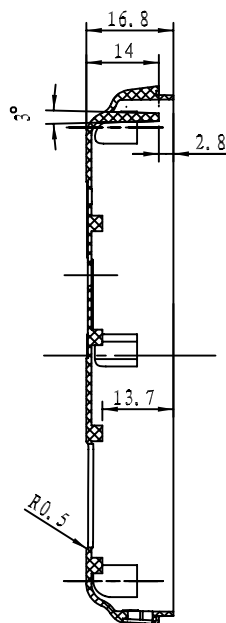
截面 B-B
