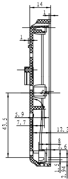
截面 C-C
