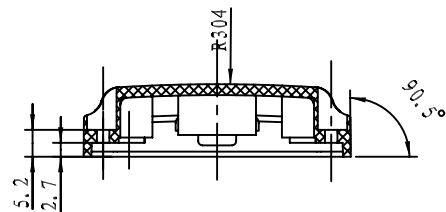
截面 A-A
