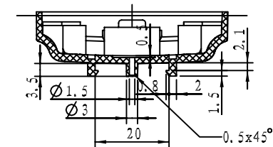
截面 B-B
