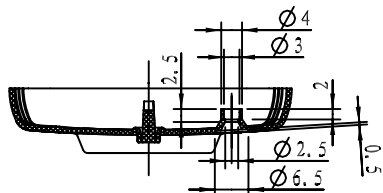
截面 B-B
