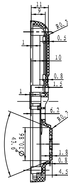
截面 A-A
