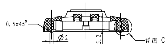
截面 C-C
