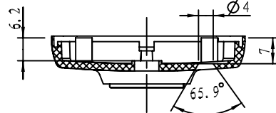
截面 B-B
