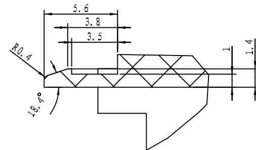
细节 A 比例 5:1
