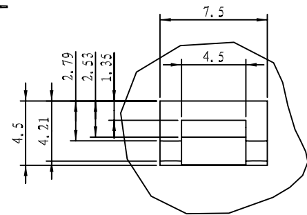
细节 D 比例 4:1
