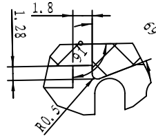
细节 G 比例 3:1
