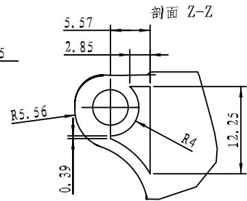
剖面 Z-Z 细节 B 比例 2:1
