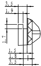
细节 F 比例 2:1
