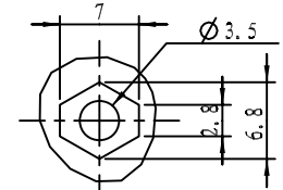
细节 C 比例 2:1
