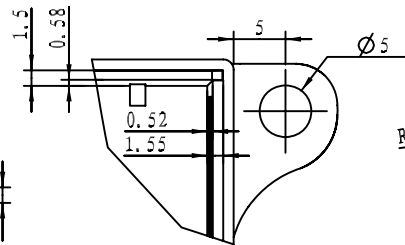
细节 A 比例 2:1
