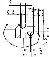
细节 E 比例 2:1
