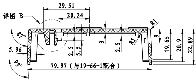
剖面 B-B
