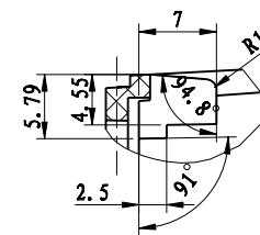
细节 A 比例 2:1
