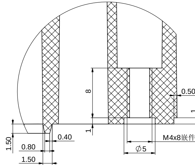
局部视图 C 比例 4:1
