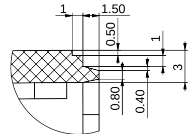
局部视图 D 比例 4:1
